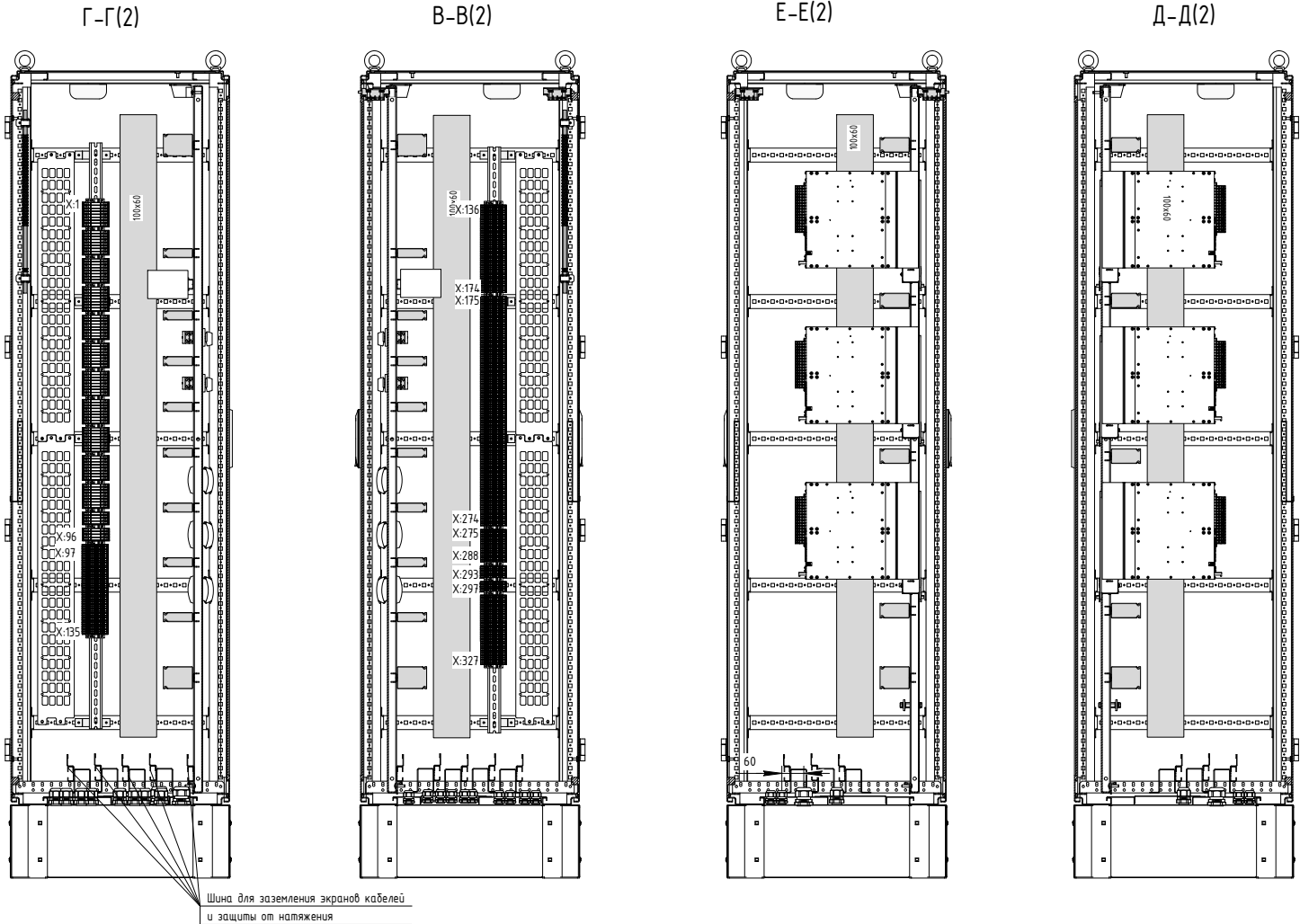
Рисунок Б.3 – Чертеж общего вида (часть 3)
