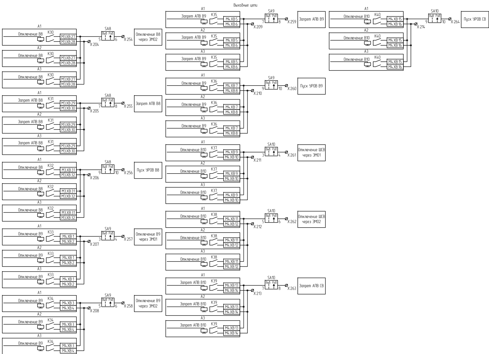
Рисунок В.10 – Схема электрическая принципиальная (часть 10)
