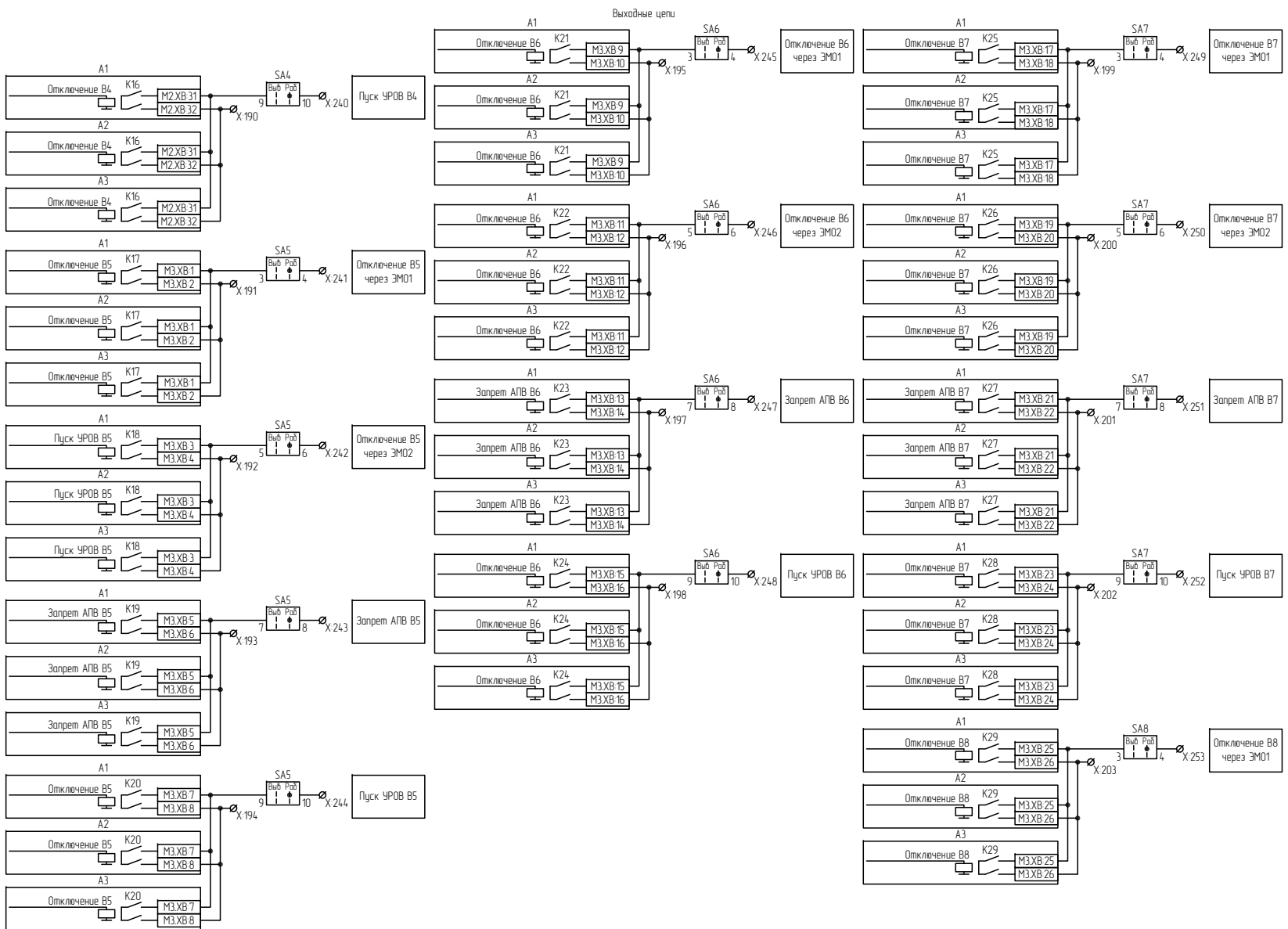
Рисунок В.9 – Схема электрическая принципиальная (часть 9)
