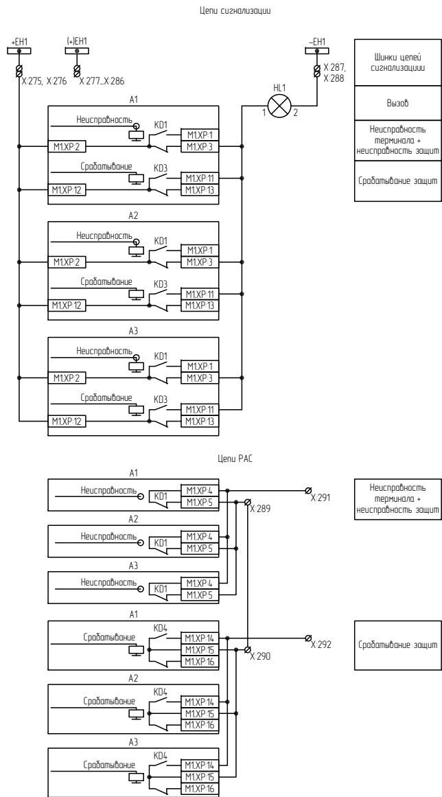
Рисунок В.11 – Схема электрическая принципиальная (часть 11)
