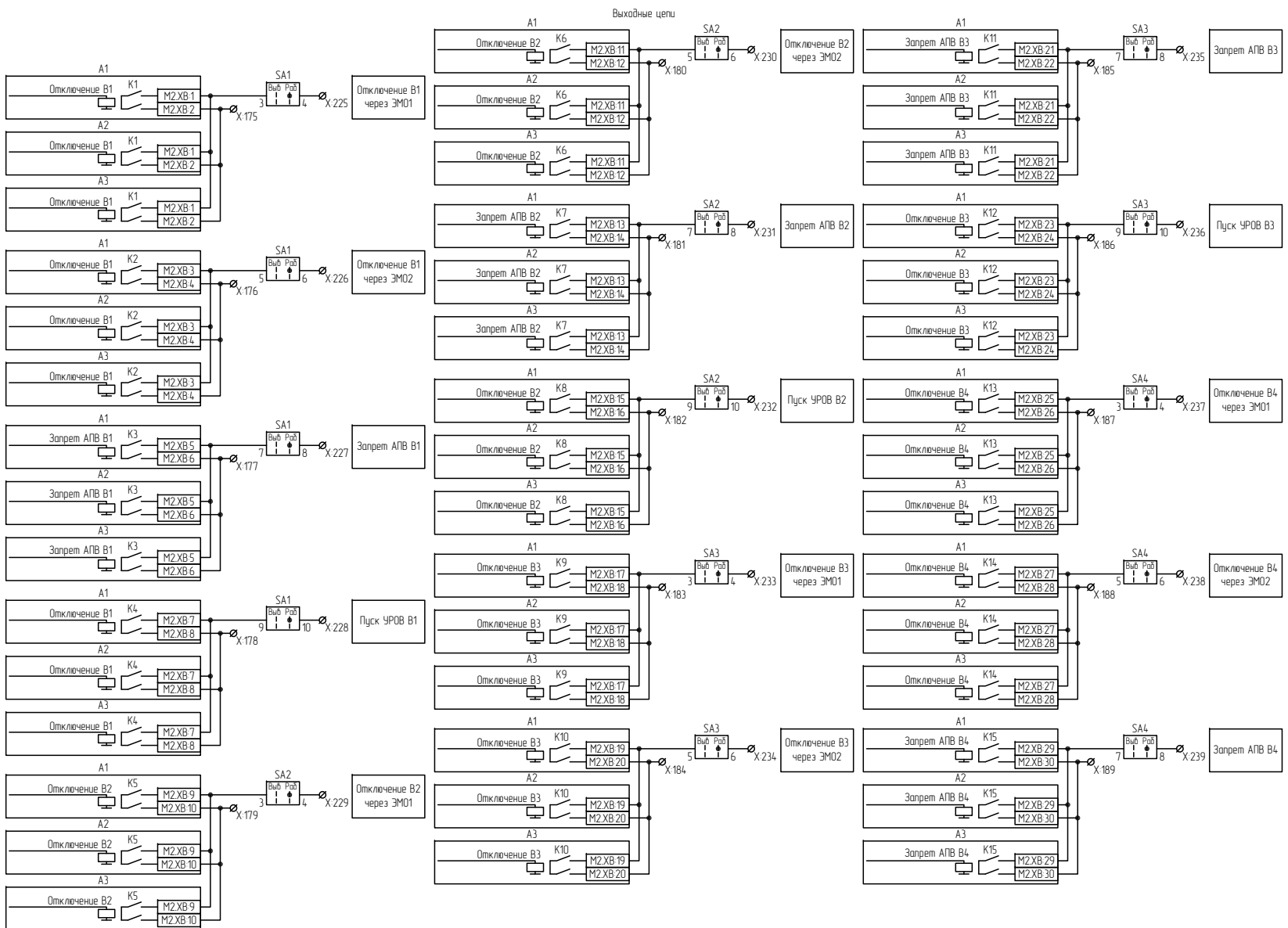
Рисунок В.8 – Схема электрическая принципиальная (часть 8)
